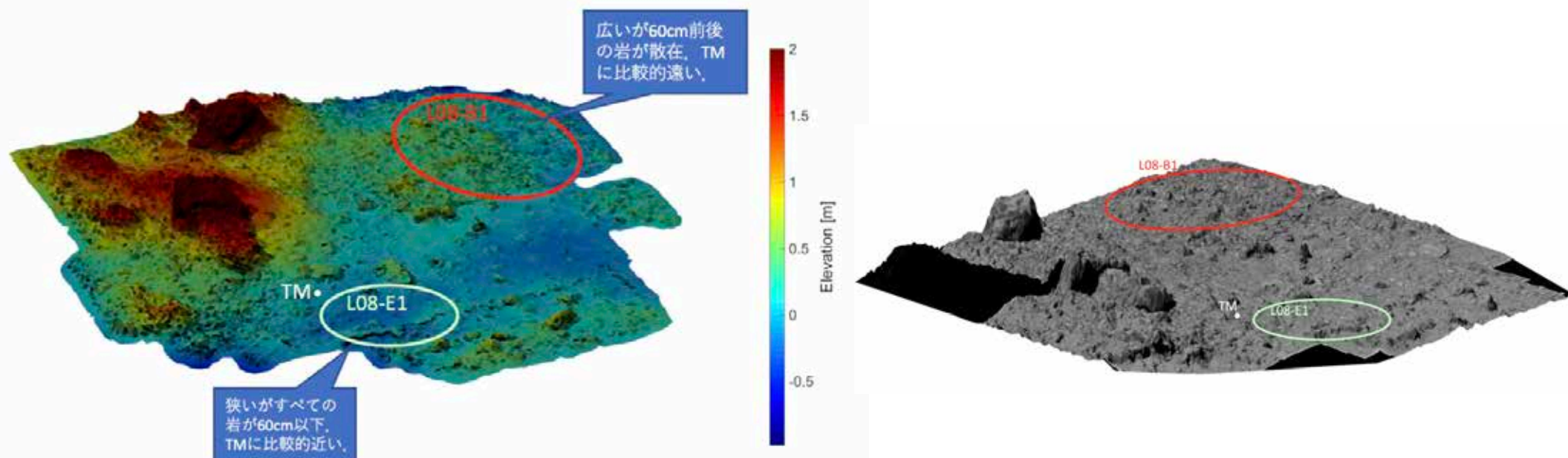
タッチダウン候補地点付近のDEM (Digital Elevation Map) (画像のクレジット: JAXA)
